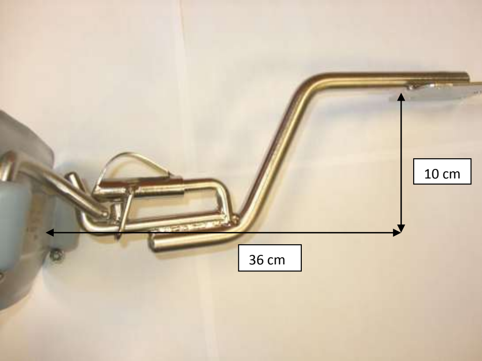
Målskisse av Weaver RBD100OS:
